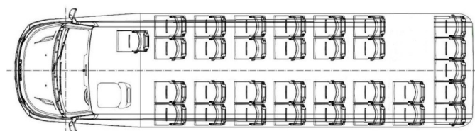
Załącznik 1 - Fotele - Układ foteli
