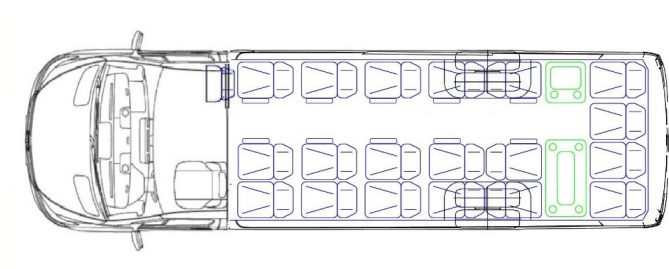
Приложение 1 - Сиденья - Расположение сидений
