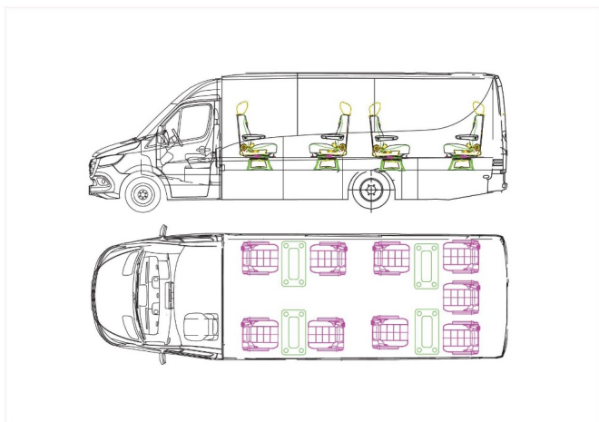
Приложение 1 - Сиденья - Расположение сидений
